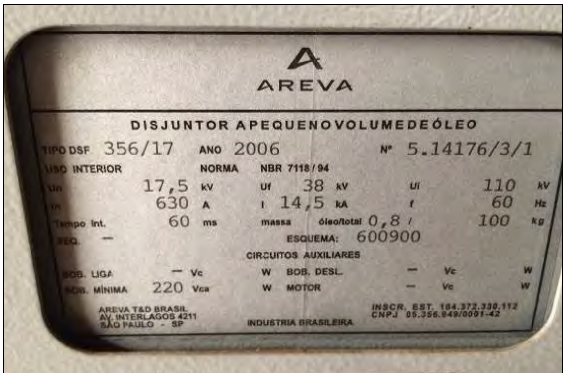
ITEM 2,213 – VISTA DA PLACA DE IDENTIFICAÇÃO DO DISJUNTOR MARCA: AREVA TIPO: 356/17 SÉRIE: 5.1476/3/1
