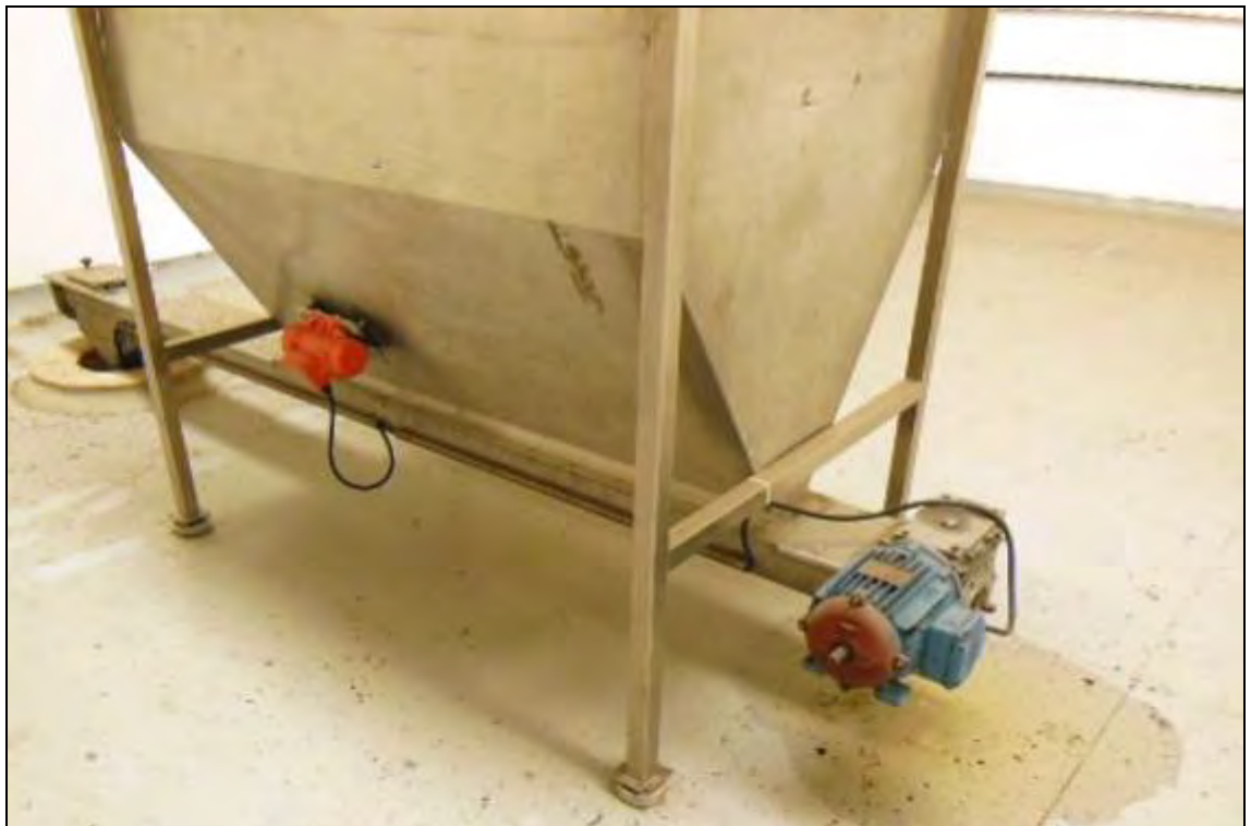
ITEM 1,034 – VISTA DO SILO FABRIMA III EM ALUMINIO COM VIBRADOR E ROSCA NA SAÍDA
