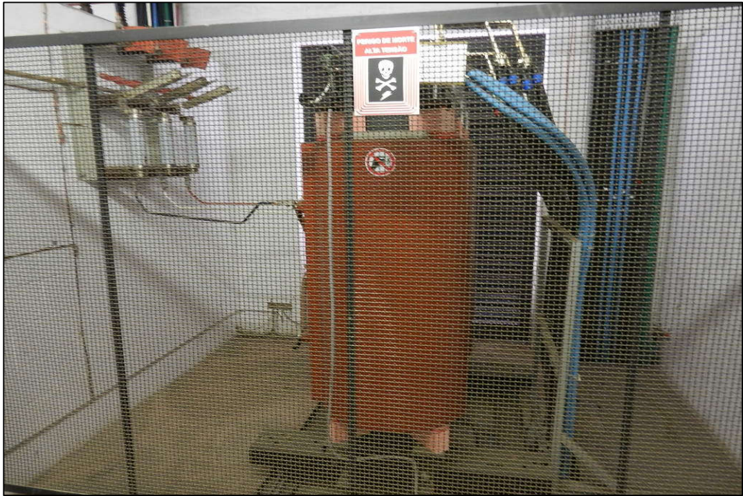
ITEM 1,153 - VISTA DA CABINE SECUNDARIA COMPREENDENDO: 1 CHAVE SECCIONADORA, 1 TRANSFORMADOR A SECO GEAFOL CAP: 2.000 KVA, 13,8/380/220V, 1 CHAVE SECCIONADORA, 1 TRANSFORMADOR MARCA: TRAF0 TIPO: TEC-1500/1.5/1.2 CAP: 1.500 KVA, 13,8/460/265,6 KV
