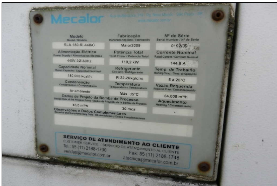
ITEM 1,129 / 1,130 - VISTA DO CONDENSADOR DE AR MARCA: MECALOR MODELO: RLA-180-RA-440/C SERIE: 0192/09 (PLACA DE IDENTIFICAÇÃO)
