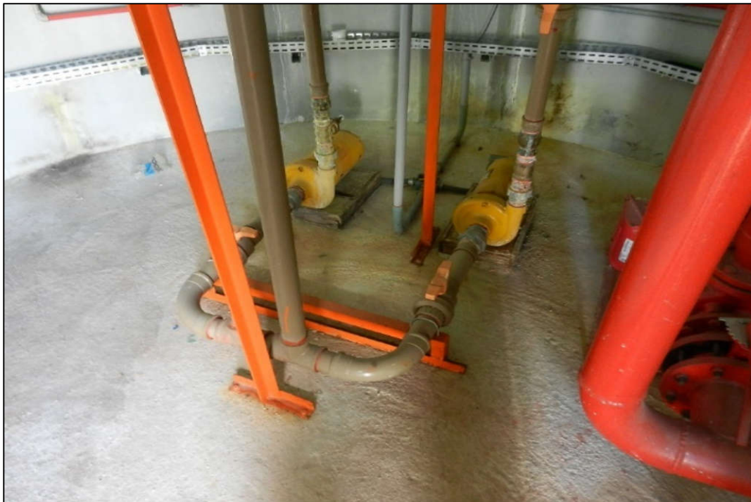
ITEM 1,131 - VISTA DAS 2 (DUAS) BOMBAS CENTRIFUGAS MARCA: JACUZZI MODELO: 3DM 1.1/2 COM MOTOR ELETRICO DE 3 CV
