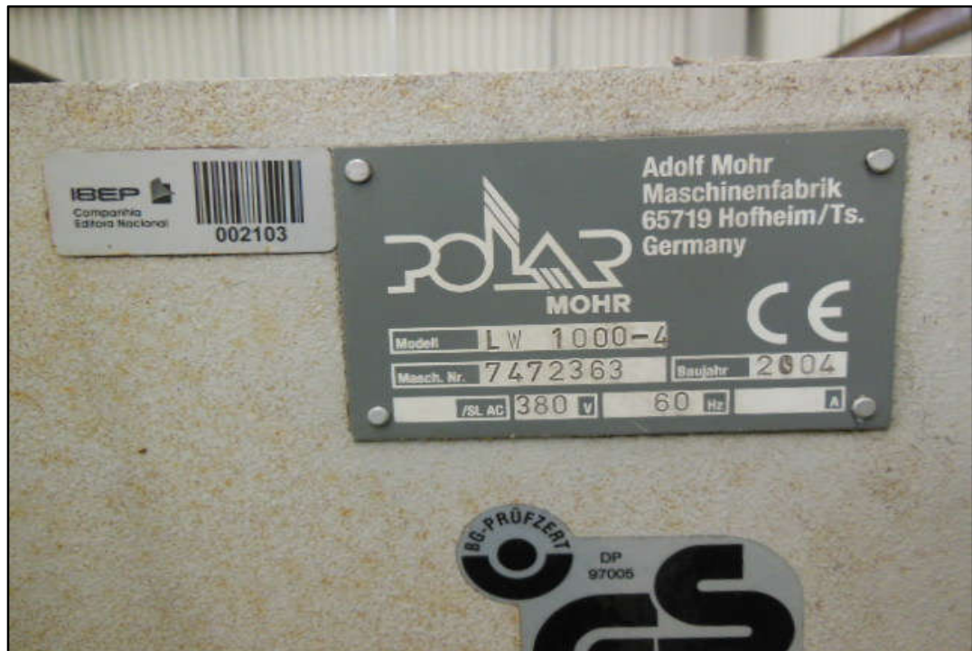
ITEM 1,016 - VISTA DA PLACA DE IDENTIFICAÇÃO DA PLATAFORMA ELEVADORA DE PAPEL MARCA: POLAR MODELO: LW 1004 EV SÉRIE:7472363
