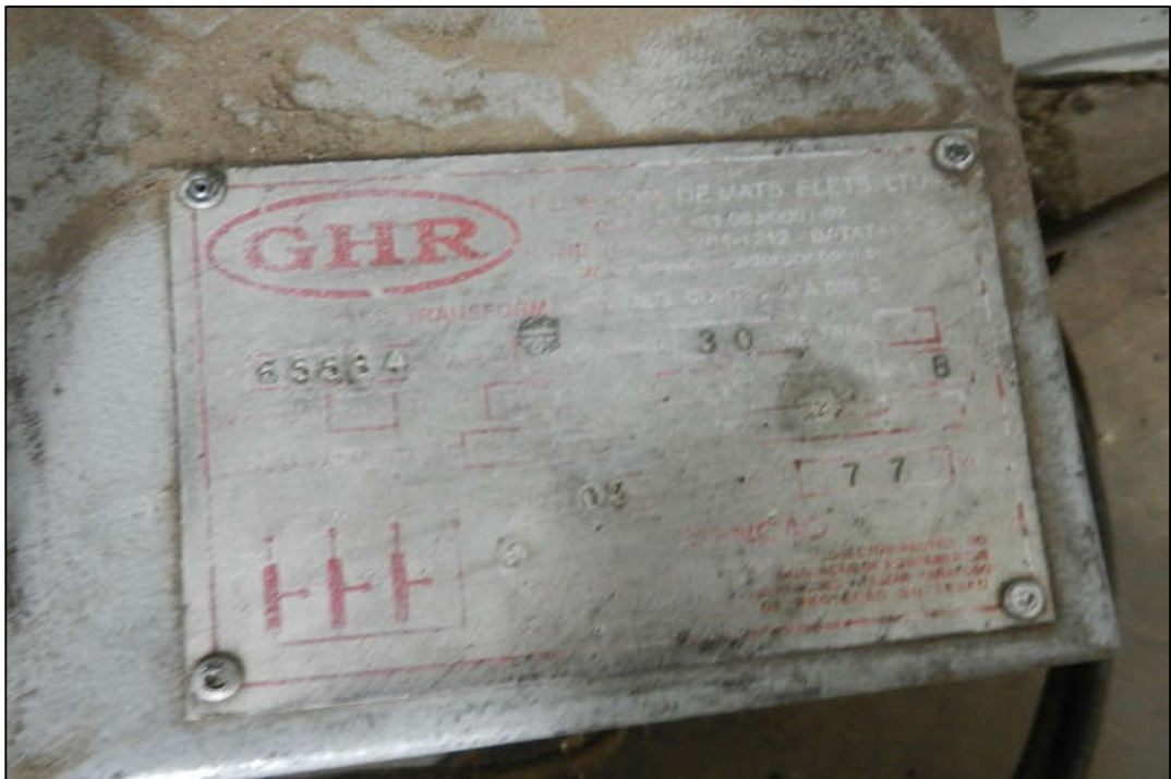
ITEM 1,117 - VISTA DO TRANSFORMADOR REG CONTINUO A SECO MARCA: GHR Nº 65.584 CAP: 30 KVA (PLACA DE IDENTIFICAÇÃO)
