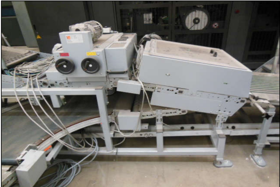
ITEM 1,033 - VISTA DA ESTEIRA (SAÍDA NA LATERAL DA GOSS) MARCA: TRANSNORM
