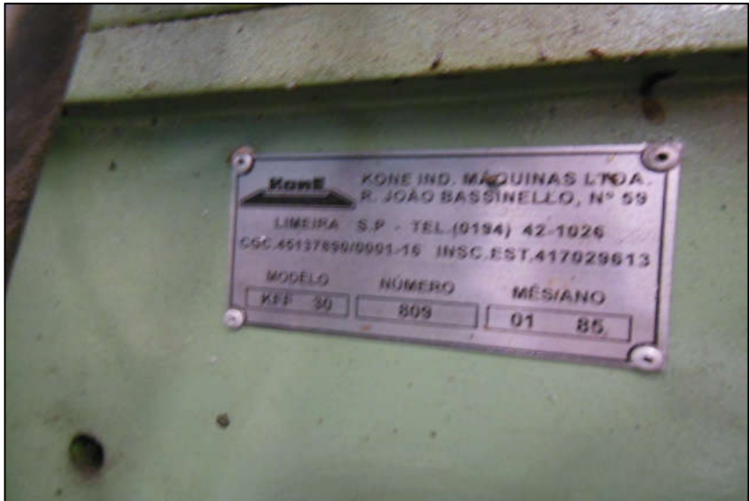
ITEM 1,056 - VISTA DA PLACA DE IDENTIFICAÇÃO DA FURADEIRA FRESADORA MARCA: KONE MODELO: KFF-30 N° 809
