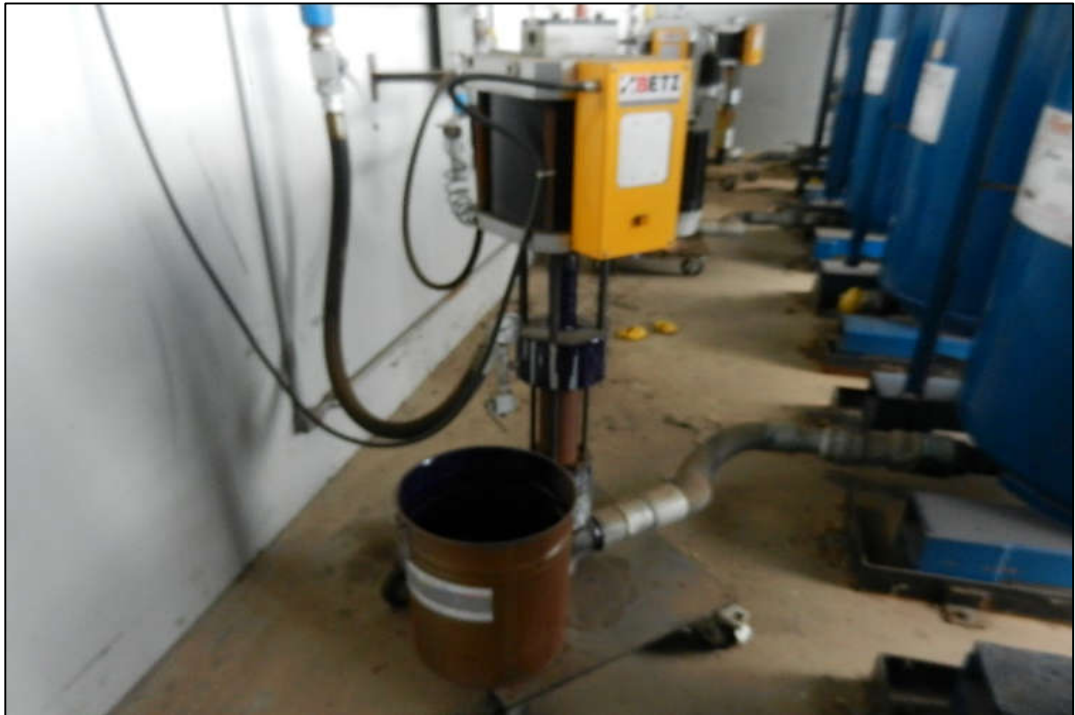
ITEM 1,122 - VISTA DAS 4 (QUATRO) BOMBAS PARA TINTA MARCA: BETZ TECNOLOGIES TIPO: P-250-1 PLC SERIES: 71210-520, 71210-518, 71210-519 E 71210-521
