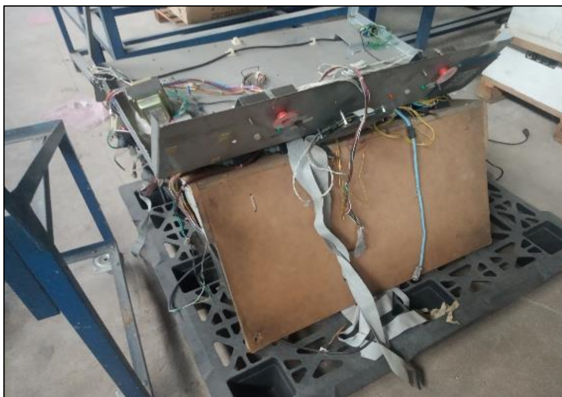
ITEM 5,010 - VISTA DO GIGA DE TESTE
