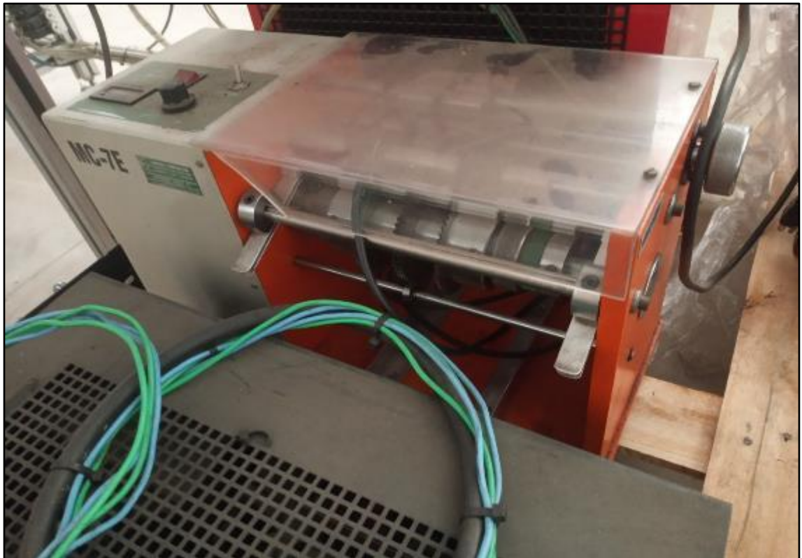
ITEM 1,026 - VISTA DA PREFOMADORA AUTOMÁTICA OMTEC MC 7E
