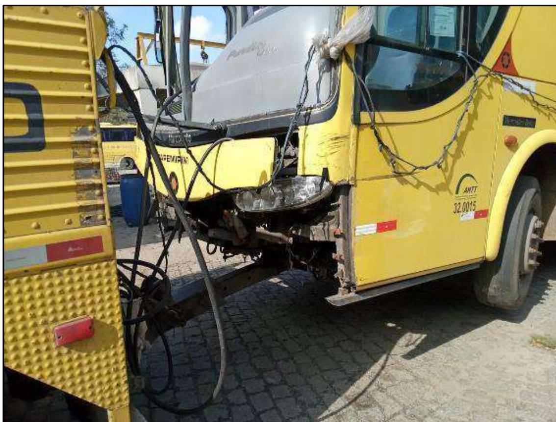
ITEM 0061 - ÔNIBUS MERCEDES-BENZ MARCOPOLO PARADISO R ANO:2008 PLACA:MSL-1260 COD:ES061
