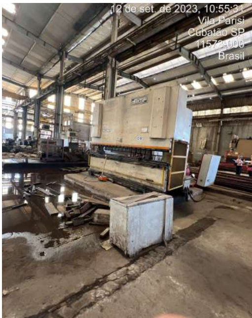
Imagem 10: Prensa dobradeira, marca NEWTON PDH 20040
