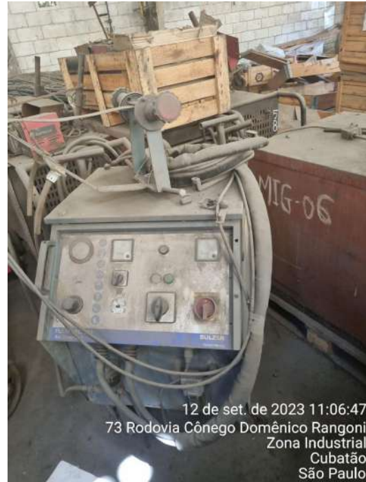
Imagem 49: Metalizadora Sulzer Flexi Arc 300
