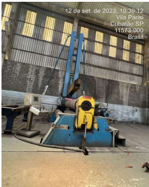
Imagem 4: Calandra de 4 Roletes, Haeusler VRM hy 3000x370
